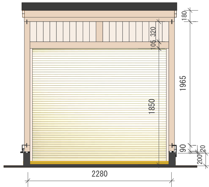
正面
