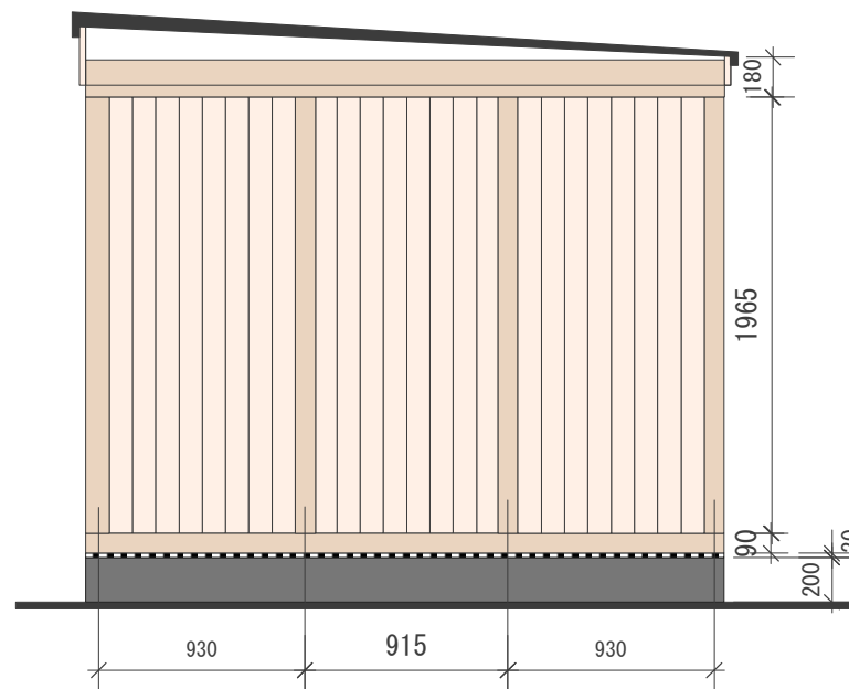
側面
