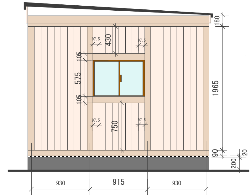
側面
